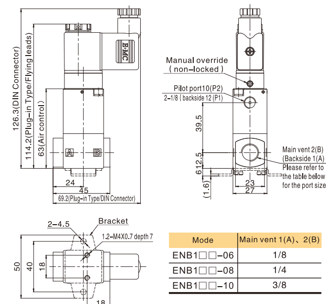
ENB1-06/08/10
