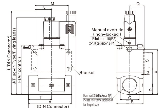
ENB2-10/15、ENB3-20、ENB4-25
